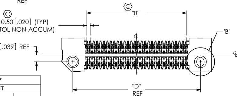
FIG 1 ERM5-030-02.0-X-DV-XX SHOWN
