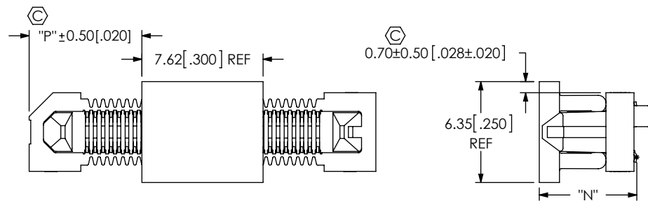
FIG 5 -P OPTION (USE PPP-08) (ERM5-030-02.0-X-DV-P SHOWN)
